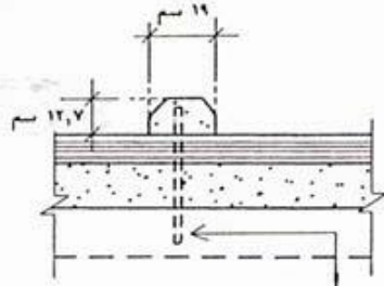
قضبان من حديد تسليح مغروسان عمودياً لتثبيت المصدرة بالأرض (العدد ١ و٢٢)
