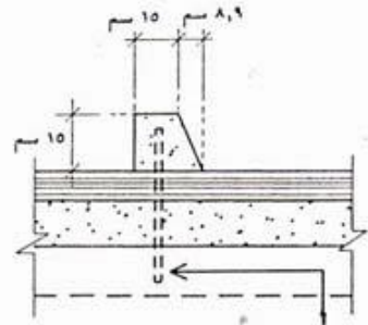
قضبان من حديد تسليح مغروسان عمودياً لتثبيت المصدرة بالأرض (العدد ١ و٢٢)
