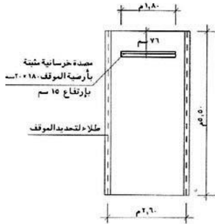
شكل رقم (٢) الحد الأدنى للمساحة المخصصة لوقوف سيارة ركاب عادية .
